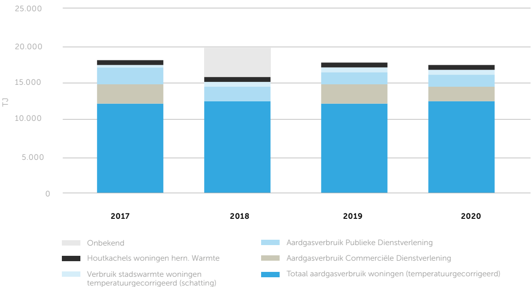
Ontwikkeling warmtevraag
