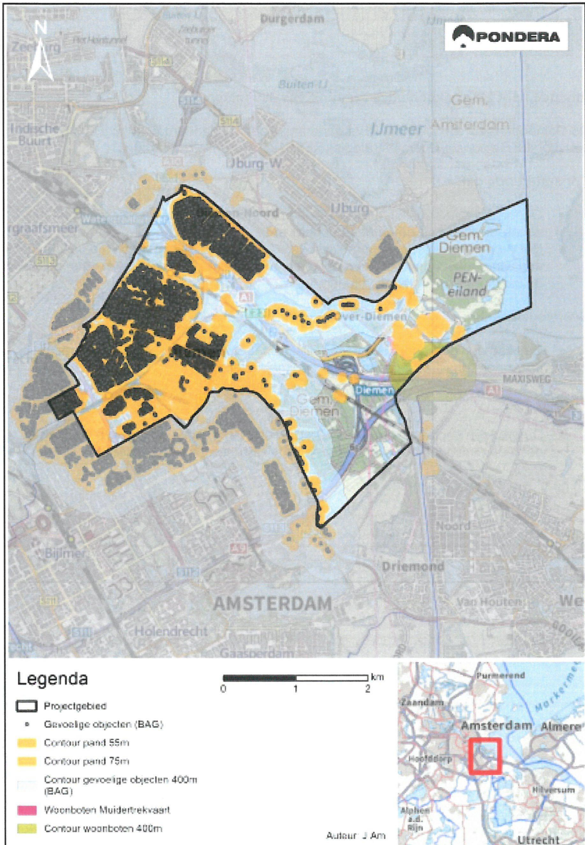
Figuur 2.1 Geluid en slagschaduwcontouren rondom de gevoelige objecten
