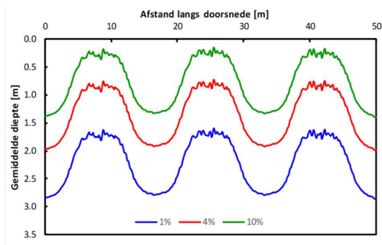
Figuur 4. Voorbeeld modelberekeningen van de diepte waarop 1%, 4% en 10% van het zonlicht op de bodem valt op een raai over drie rijen staande panelen binnen een atol. Uit Boderie & Van Aken 2022.
